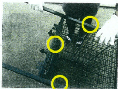
④ 金網を手前に引き、アングルの溝（3箇所）に金網を重ねないように入れてかぶせます （重要な作業です）
