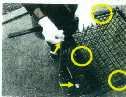
⑤蝶ネジをしっかりと締め付けます 金網が3か所の溝に（○印）入っているか確認してください
